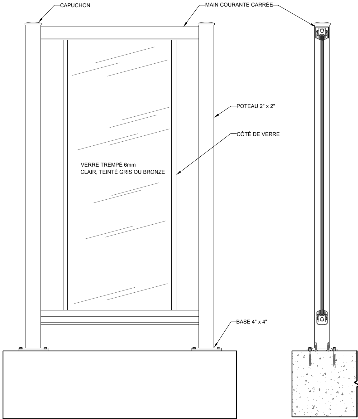
ÉLÉVATION
