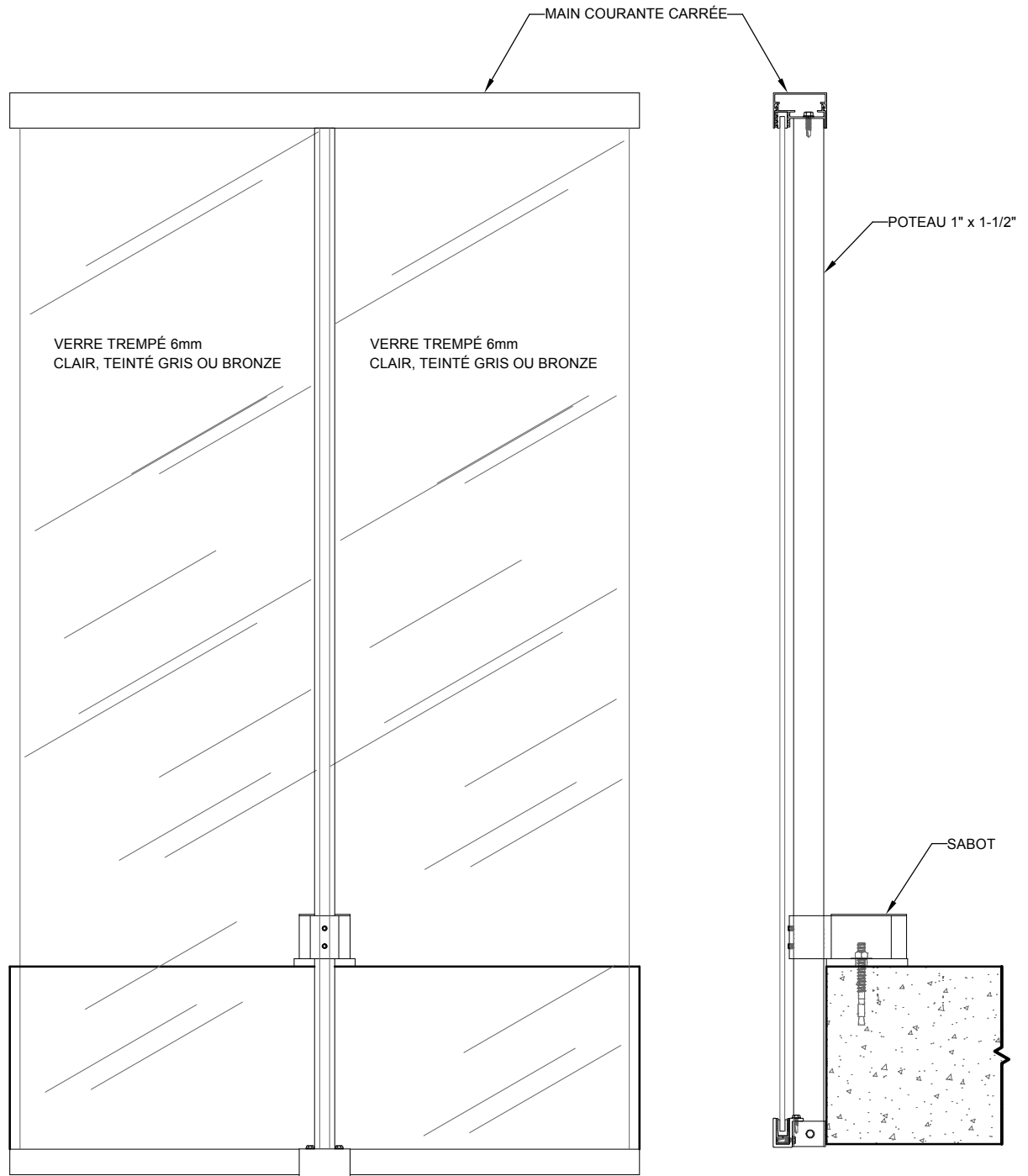
COUPE
